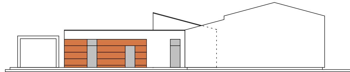
POHLED SEVEROVÝCHODNÍ
