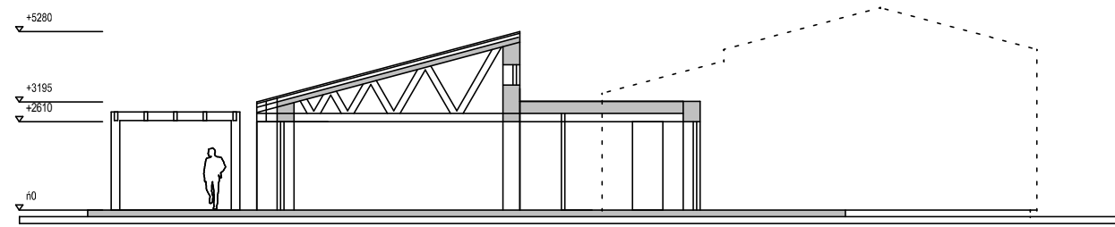
REZ PŘÍČNÝ
